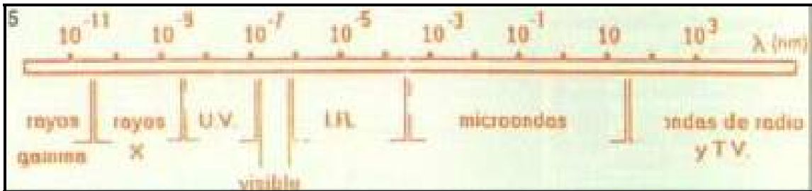
Fig. 5. Regiones del espectro electromagnético. Se indican las longitudes de onda correspondientes a cada tipo de radiación.
