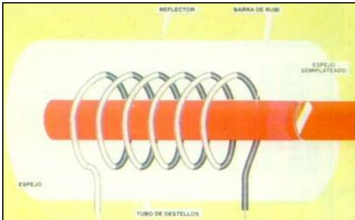
Fig. 6. Esquema interno de un láser sólido de rubí, cuyas características son similares a las de uno de gas o líquido.
