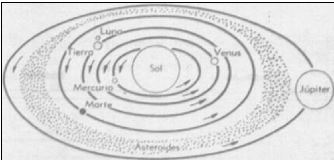
Fig 2. Los electrones giran alrededor del núcleo, como hacen los planetas en torno al Sol.
