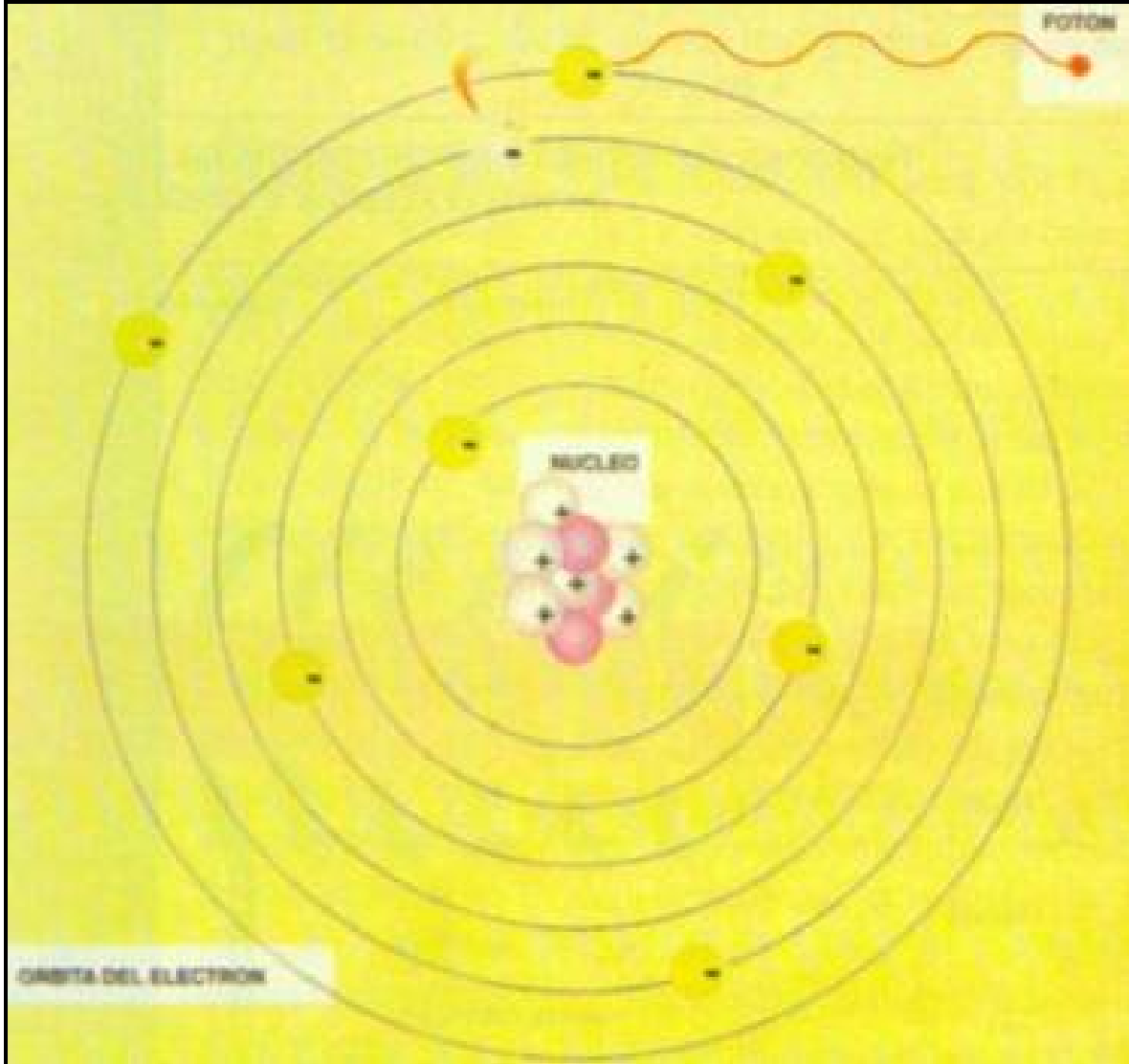
Fig. 3. La distribución de las partículas que forman el átomo.
